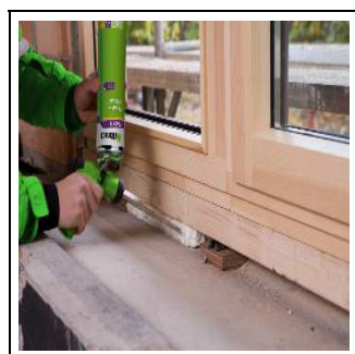
1. Bild: Verarbeitung der Fensteranschlussfuge mit FM220.
