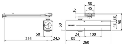
Maßzeichnungen
