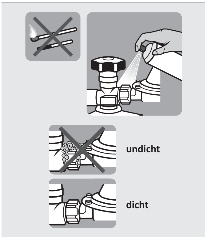
Abb.2: Dichtheitsprüfung
