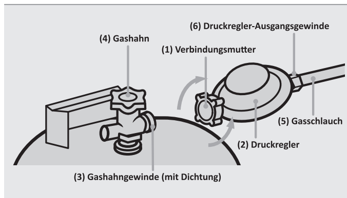
Abb.1: Montage des Druckreglers
