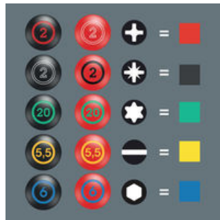
Schraubendreher Take it easy: Farbkennzeichnung nach Profilen und Größenstempelung.
