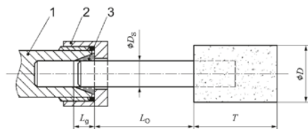
Rys. 1: Długość mocowania uchwytu zaciskowego i zacisku
