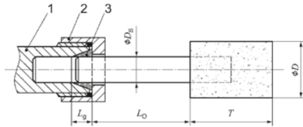
Resim 1: Gerdirmе aynası ile gerdirmе pensi arasındaki gerdirmе uzunluğu Açıklamalar
