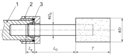
Fig. 1: Inspänningslängd från spännoch och spännhylsa
