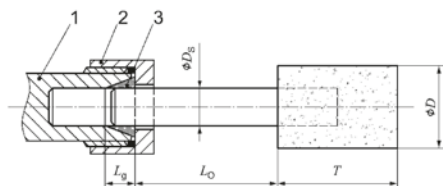
Afb. 1: spændepatronens fastspændingslængde og spændetang
