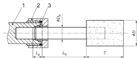
Фиг. 1: Дълбочина на захвата на патронника и на цагата
