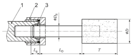
Obrázek 1: Délka upnutí skličidla a kleštíny
