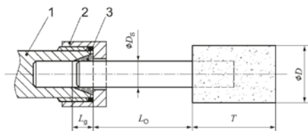
Εικόνα 1: Μήκος τοποθέτησης εργαλειοδέτη και κόλτε
