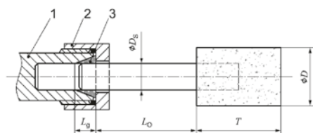
Slika 1: Dužina upregnuća zatezne čahure i zateznih klijesta
