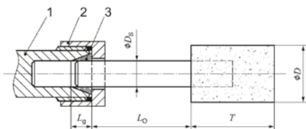
Kuva 1: Kiristinstukan ja kiristyspihdin kiinnityspituus
