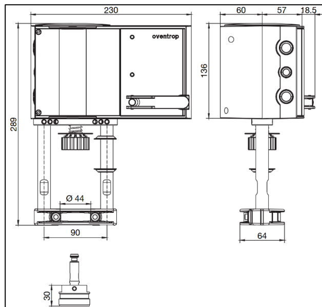
Maße der Antriebe und Anschlussmaße des Adapters
