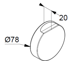
Maßzeichnung
