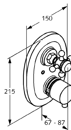
Maßzeichnung I
