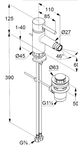
Maßzeichnung
