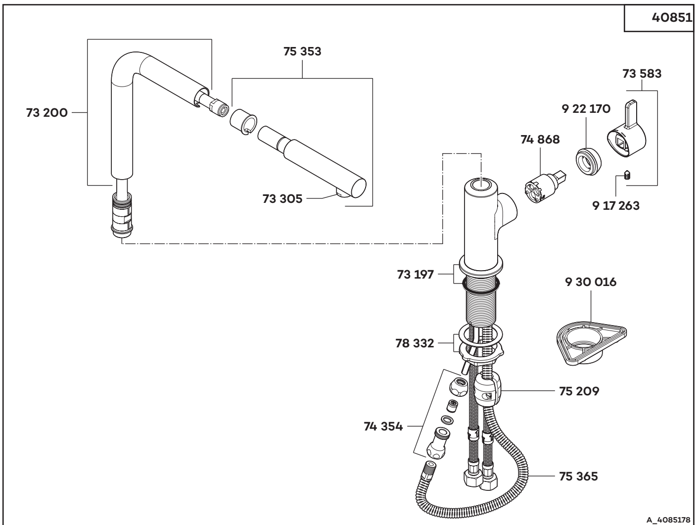
40851 Spültisch-Einhandmischer DN 15 single lever sink mixer DN 15 ééngreeps gootsteenmengkraan 1/2"
